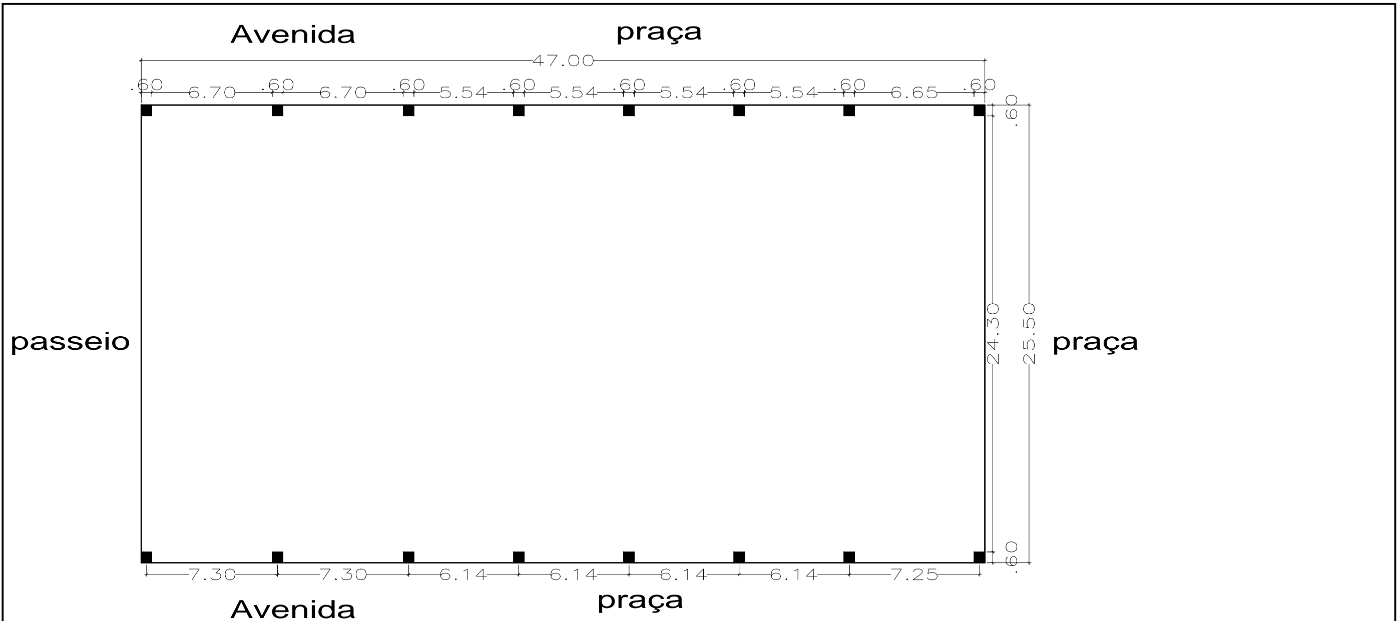
PLANTA BAIXA A: 1.198,50 m 2
